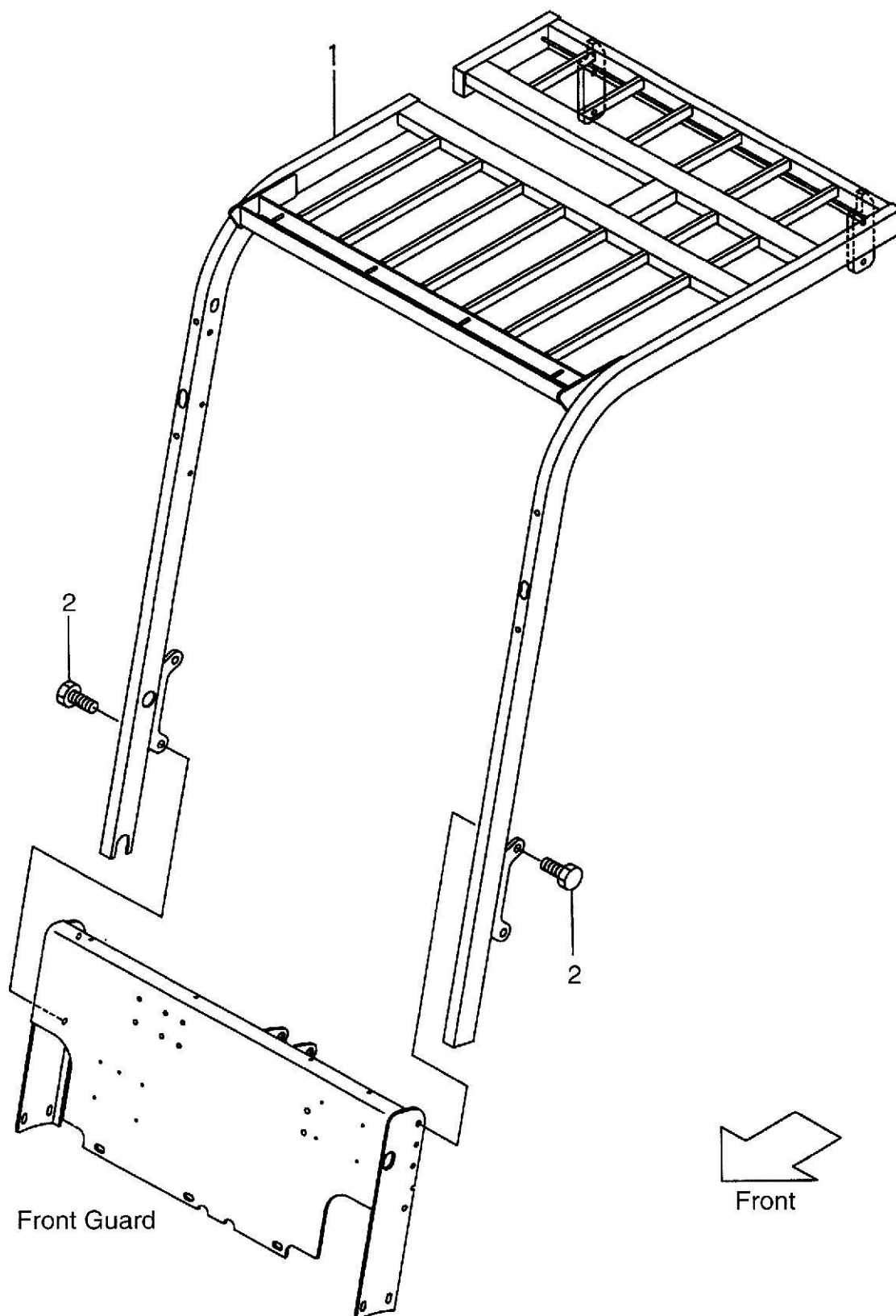
图 19 护顶架
