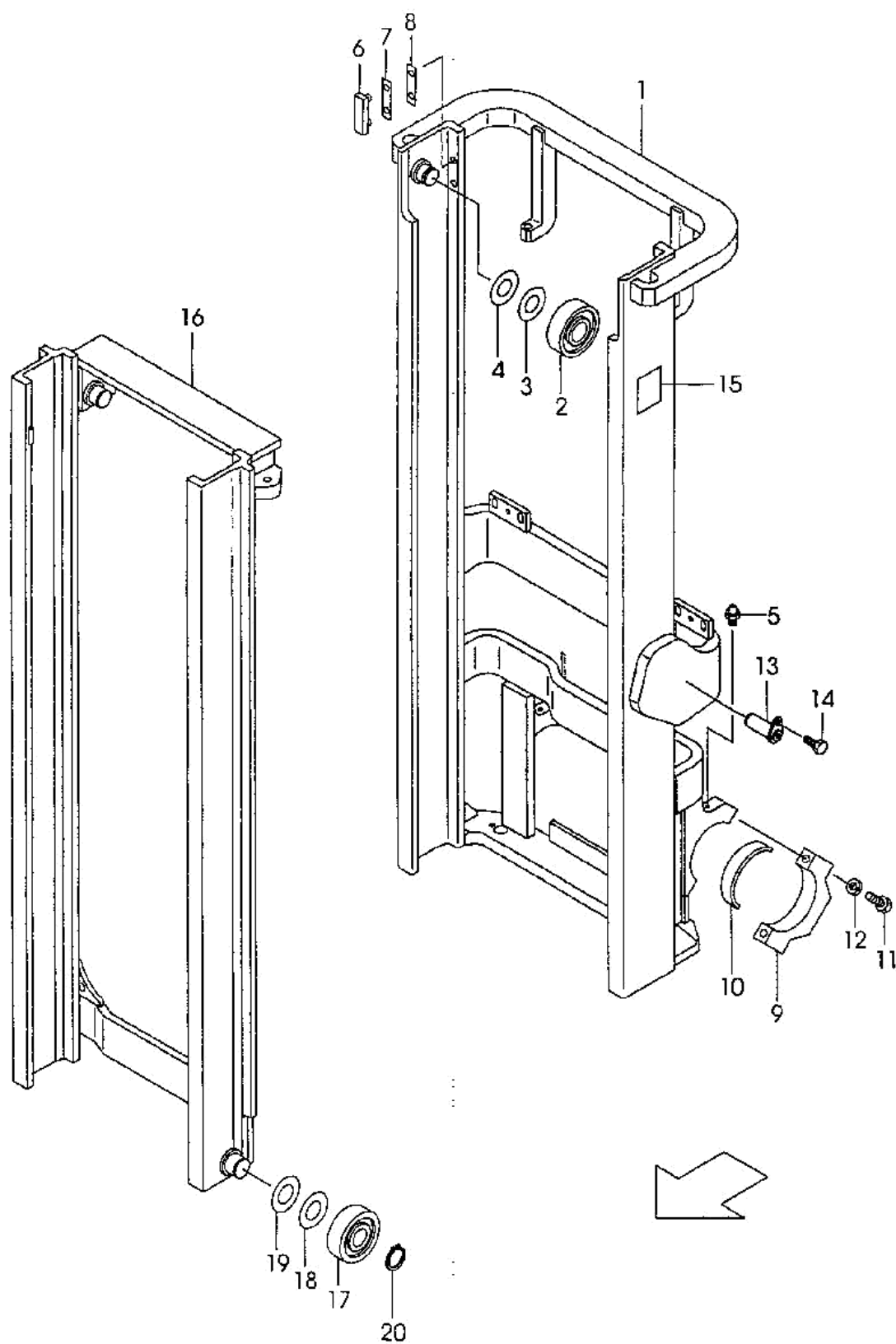
图 51-4 标准门架(EK40-VM)
