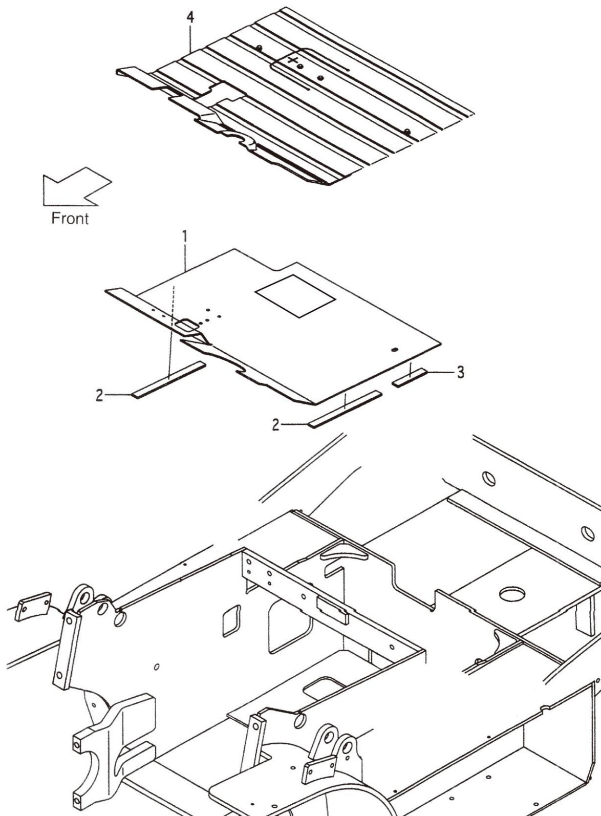
图 38 前底板
