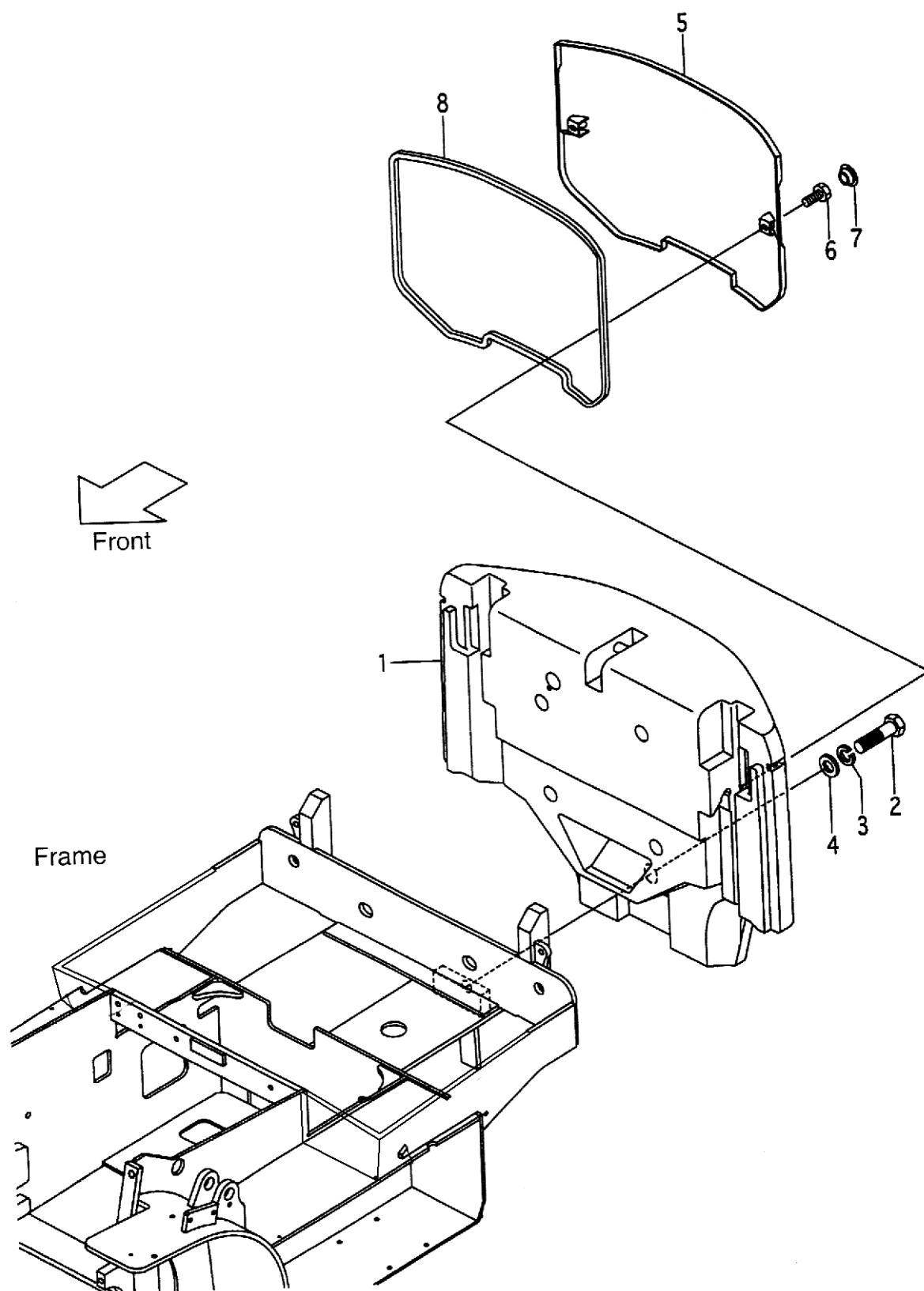
图 34 平衡重
