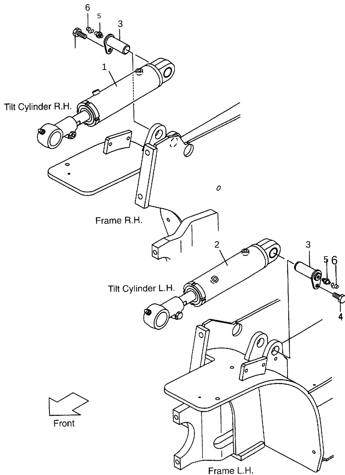
图 46-1 倾斜油缸/销
