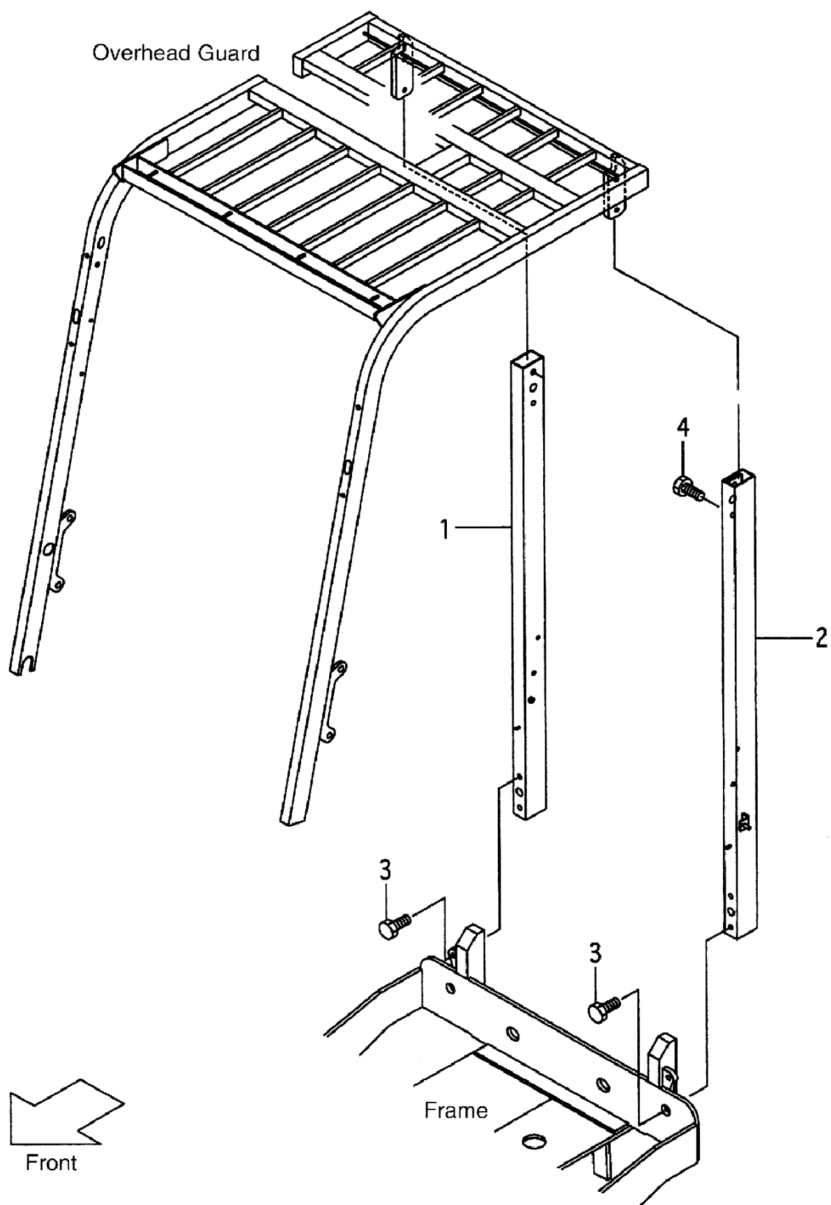
图 20 后腿
