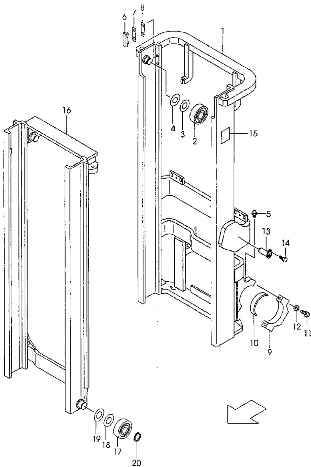
FIG.51-3 MAST [VM31E] [VM36E] 图 51-3 标准门架(EK30-35-VM)
