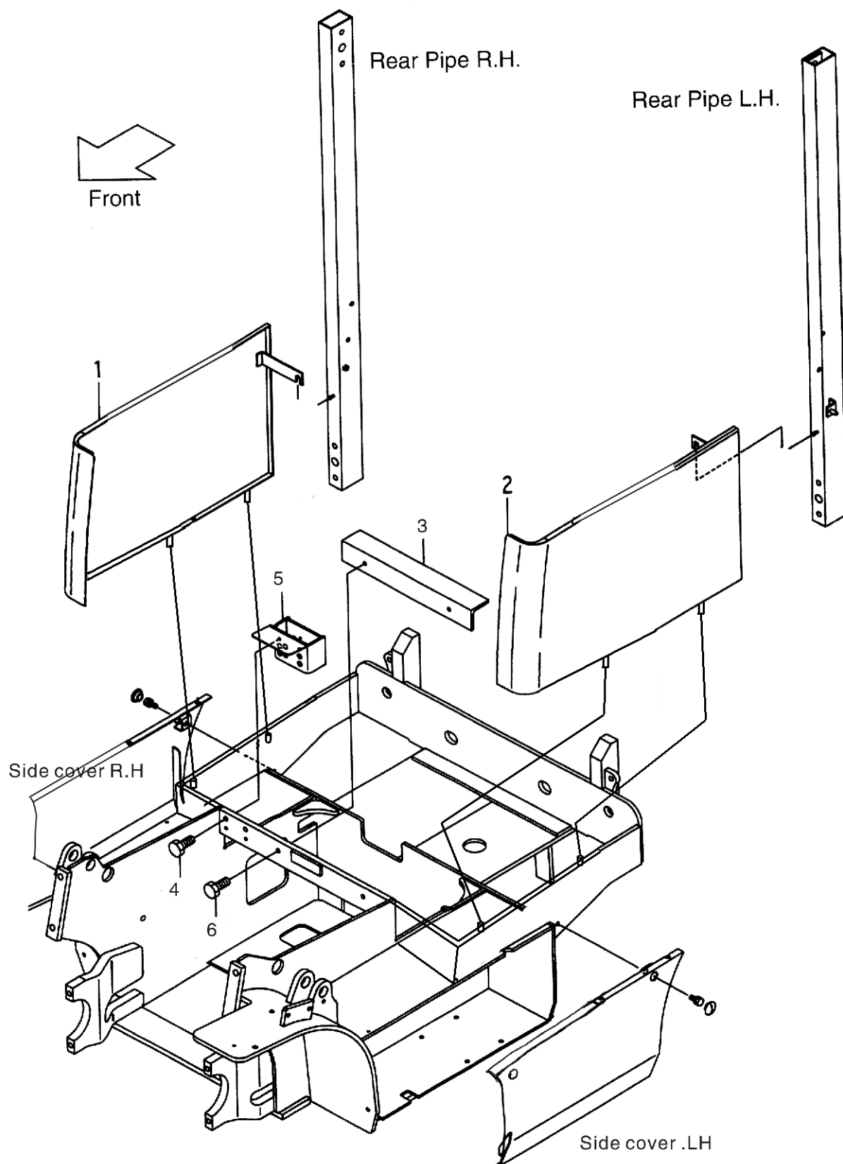
图 37 电瓶侧板
