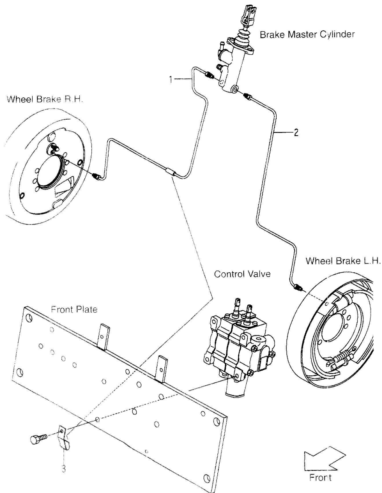
图 31 制动钢管
