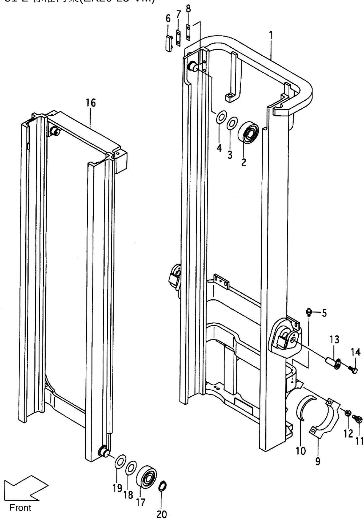
图 51-2 标准门架(EK20-25-VM)
