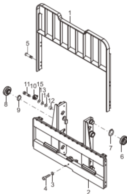
货叉架挡货架选用件表 FORK OPTIONAL PARTS
