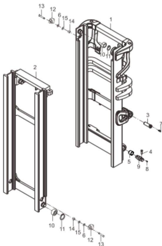
门架选用件 MAST OPTION TABLE
